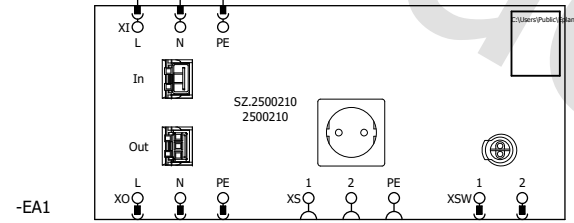
Systemleuchte LED 900, 100-240 V, L: 437 mm, mit Steckdose
